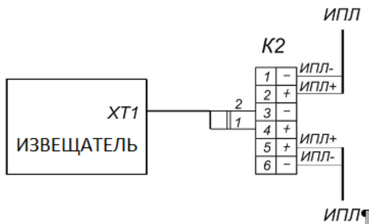
Рисунок 4–Схема подсоединения извещателя
