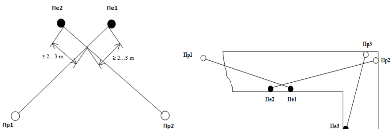
Рисунок 2 –Перекрытие секторов зоны обнаружения
